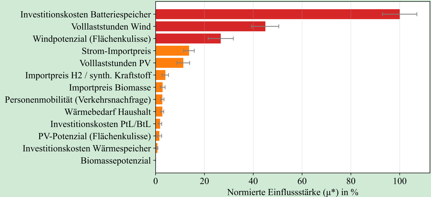
3. Unsicherheit Optimierte Stromspeicher-Kapazität aus 1,400 Simulationen
