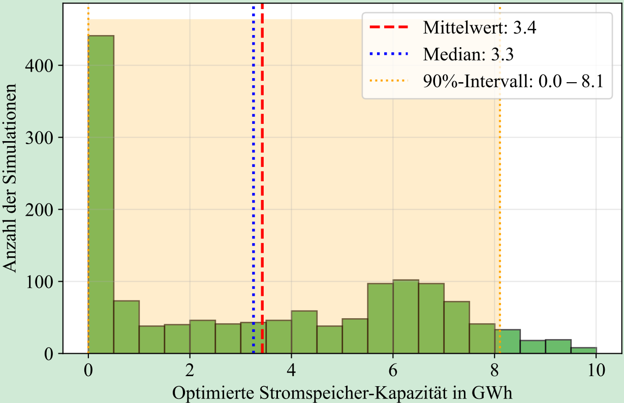
3. Unsicherheit Optimierte Stromspeicher-Kapazität aus 1,400 Simulationen
